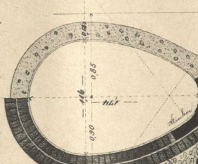
Querschnitt Prof. 155 qm
