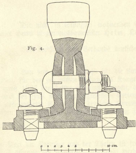
Fig. 4 und 5. Zahnstange.
