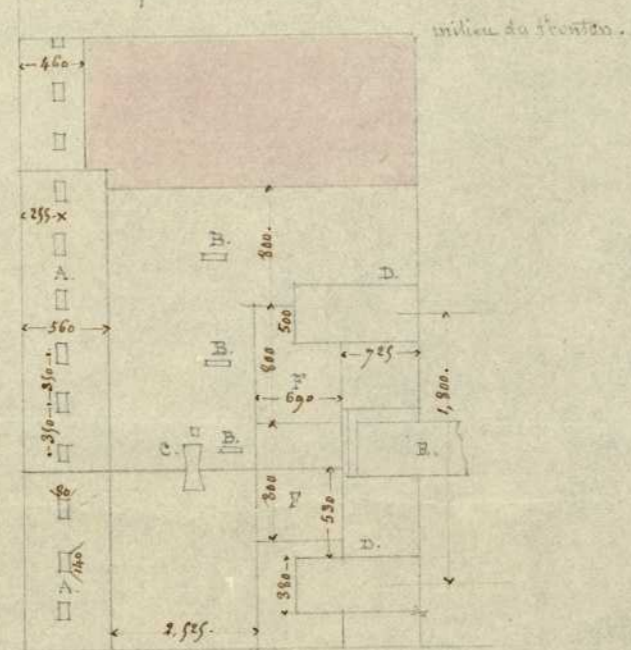
Plan d'une partie du dessus du Fronton.
