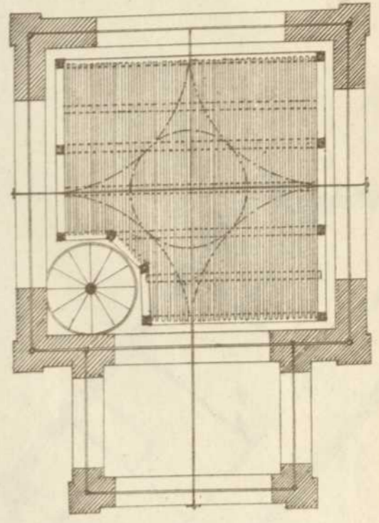
Grundriss des Baderaus mit Lattenrost.
