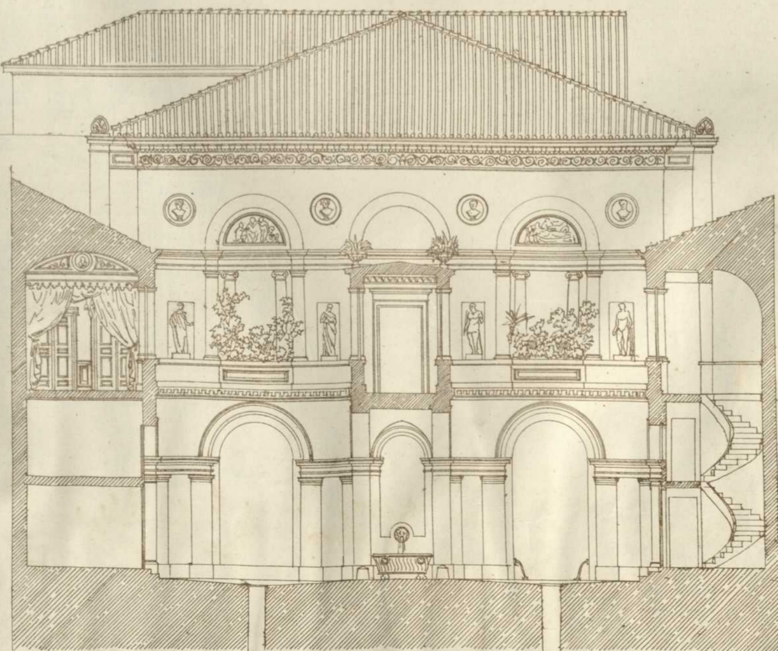
Quer-Schnitt.
