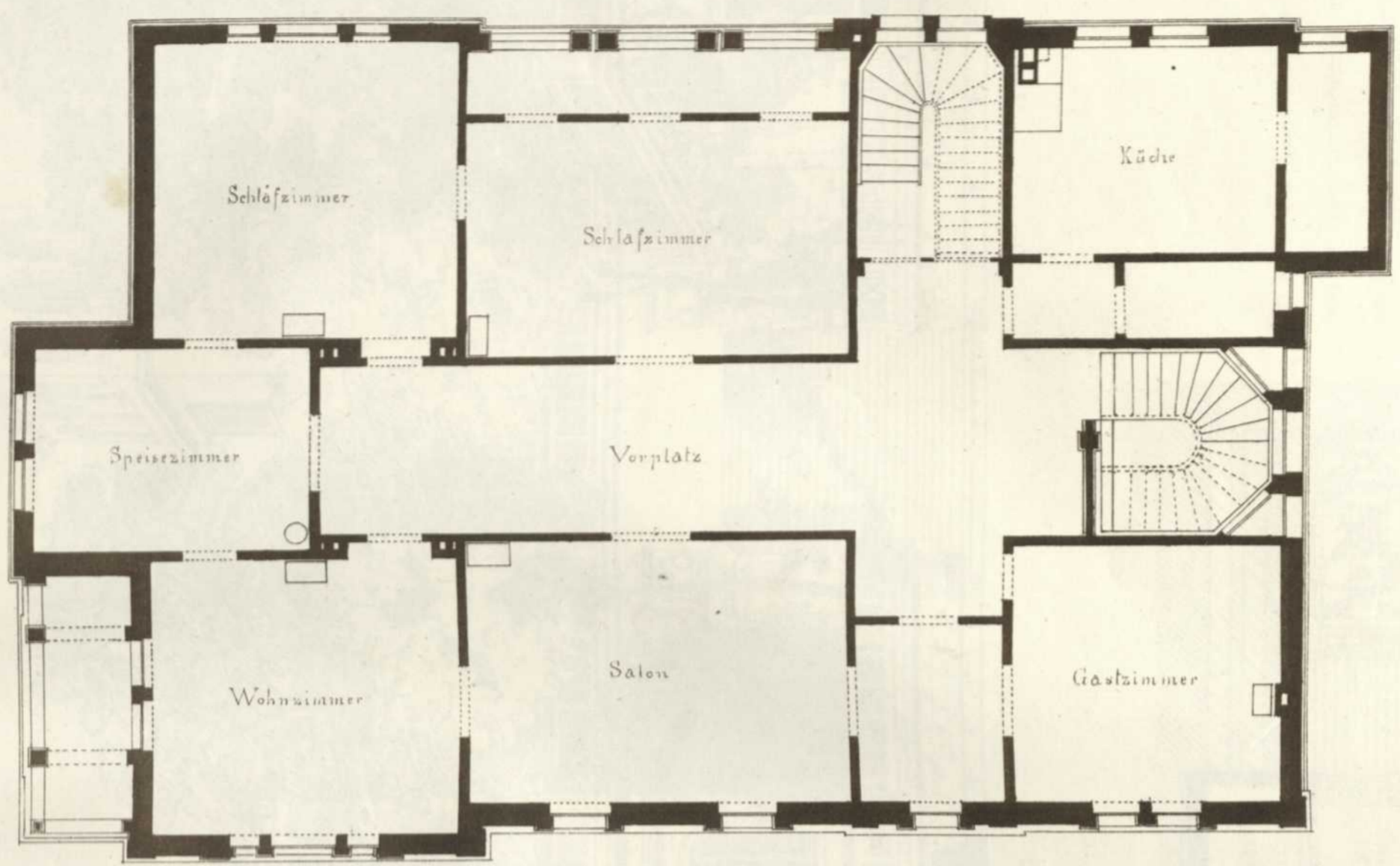
Grundriss des obern Stocks.
