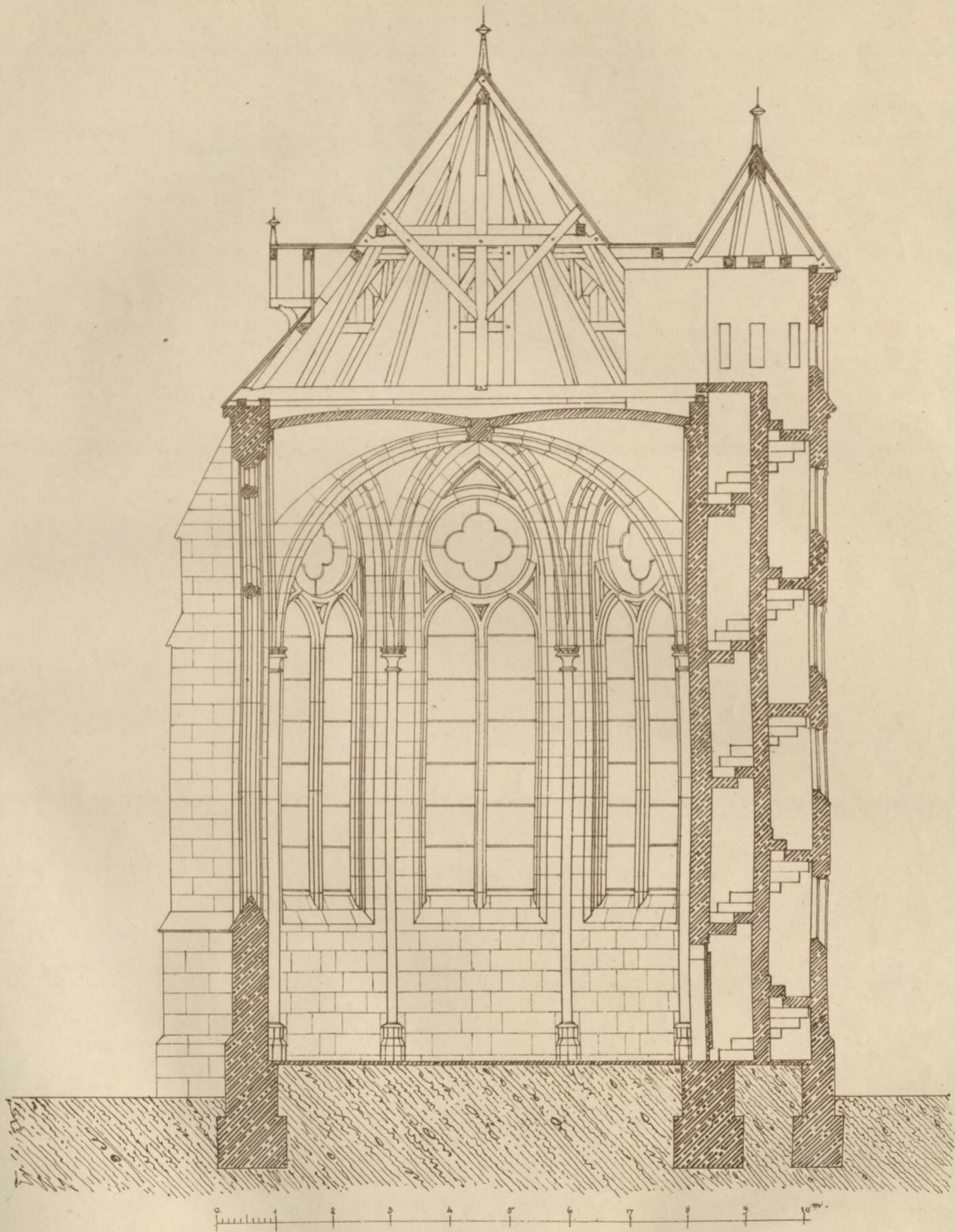
Durchschnitt durch die Kapelle nach a-b.
