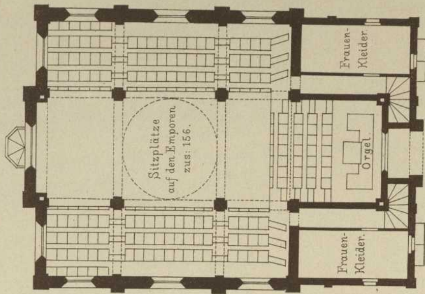
Grundriss der Emporen.
