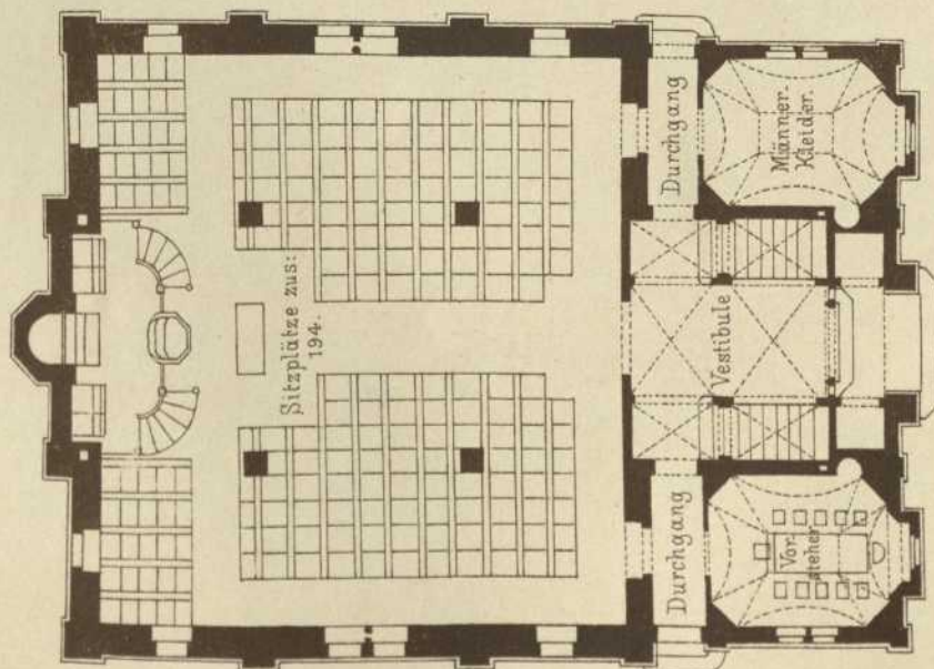
Grundriss zu ebener Erde.
