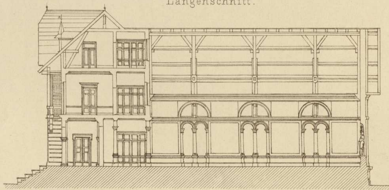
Längenschnitt.
