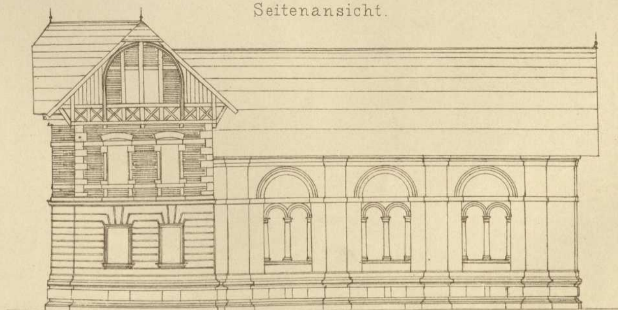
Seitenansicht.
