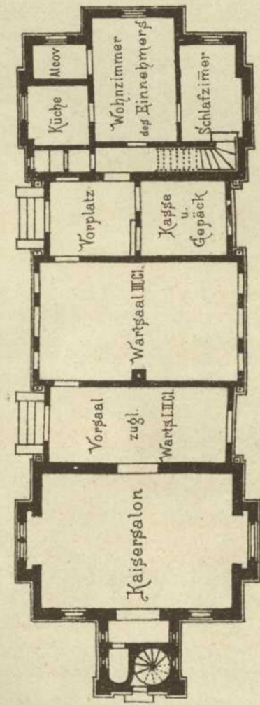
Grundriß des Parterre.
