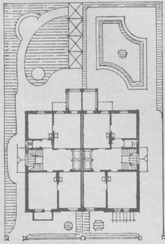
Fig. 6. (Doppelhaus.)
