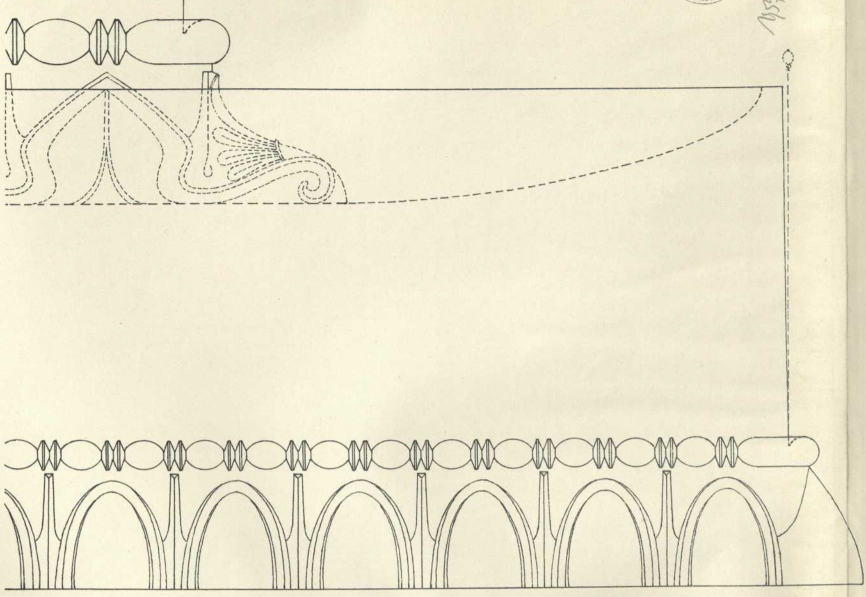
Fig. 5. Kranzplatte des Nordportikus \frac{1}{2} n. Gr.
