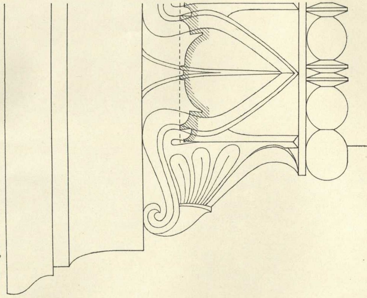
Fig. 4. Architravgesims am Nordportikus n. Gr.
