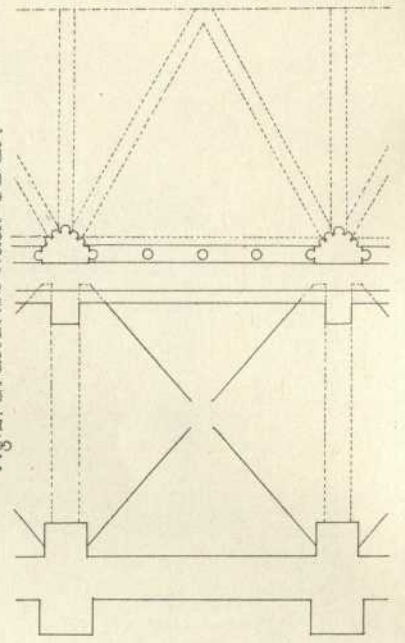
Fig. 2 Grundriss nach C'D'E'F.
