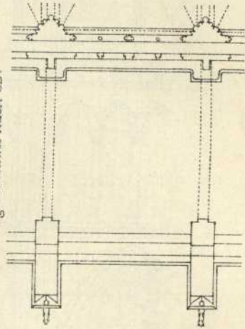
Fig. 2. Schnitt nach CD.
