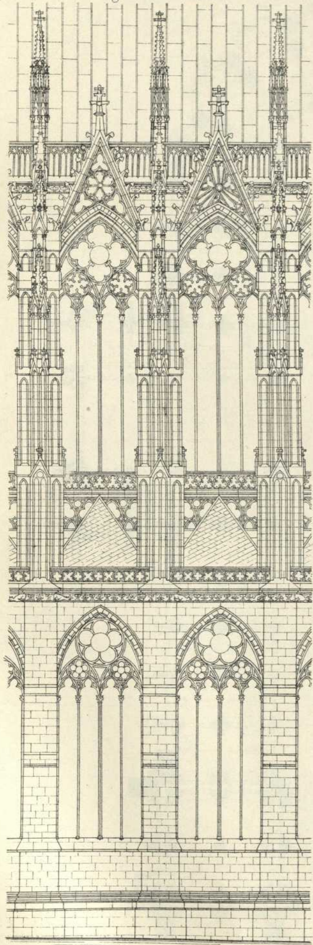
Fig 2. Aussenansicht.
