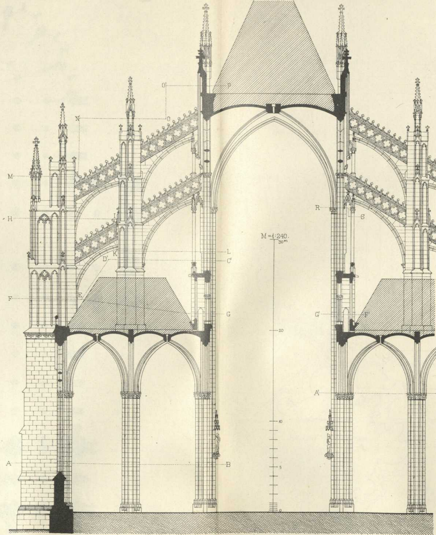
Fig 4 Querschnitt.
