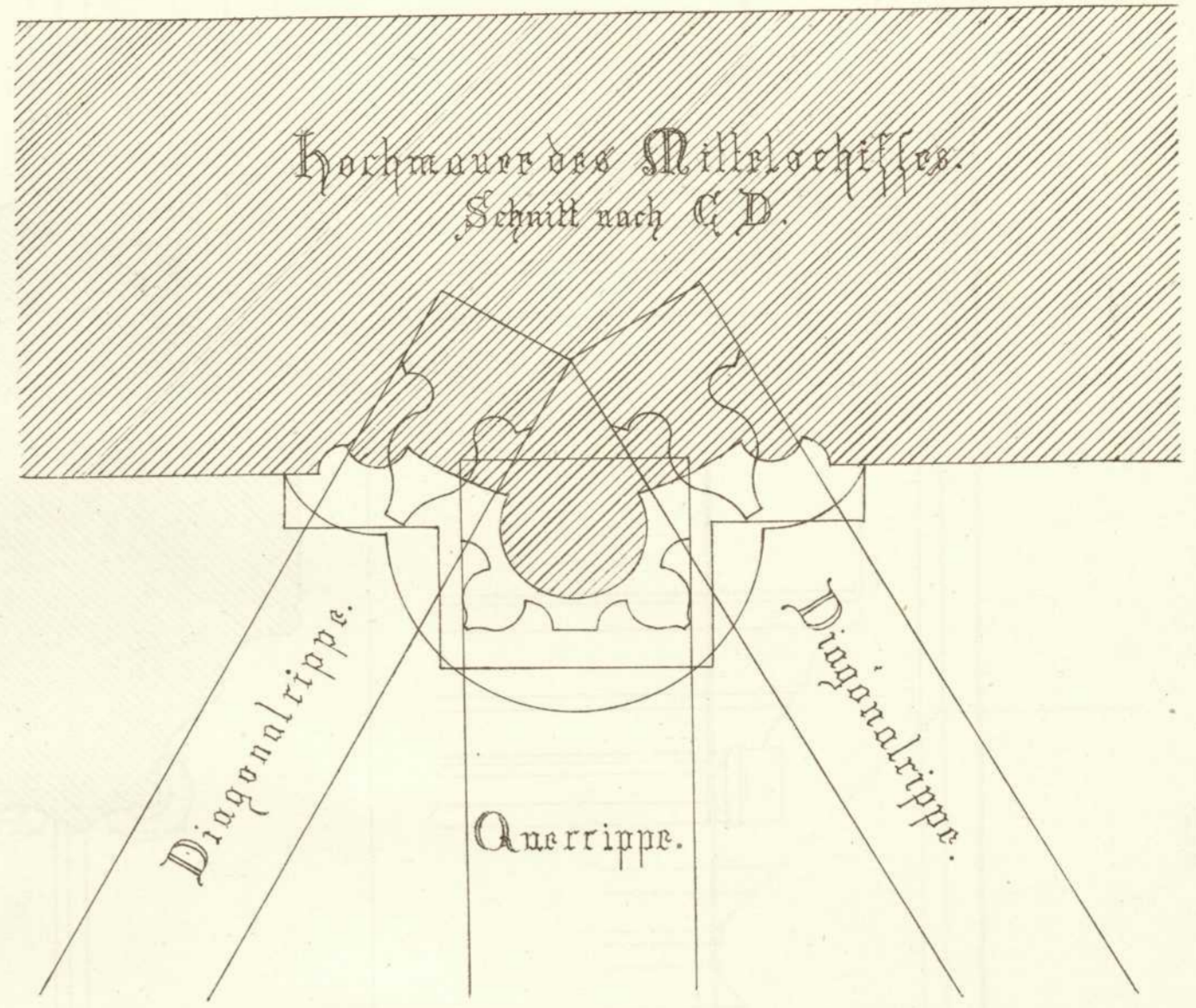
Grundriß der Gewölbanfänge des Mittelschiffes.
