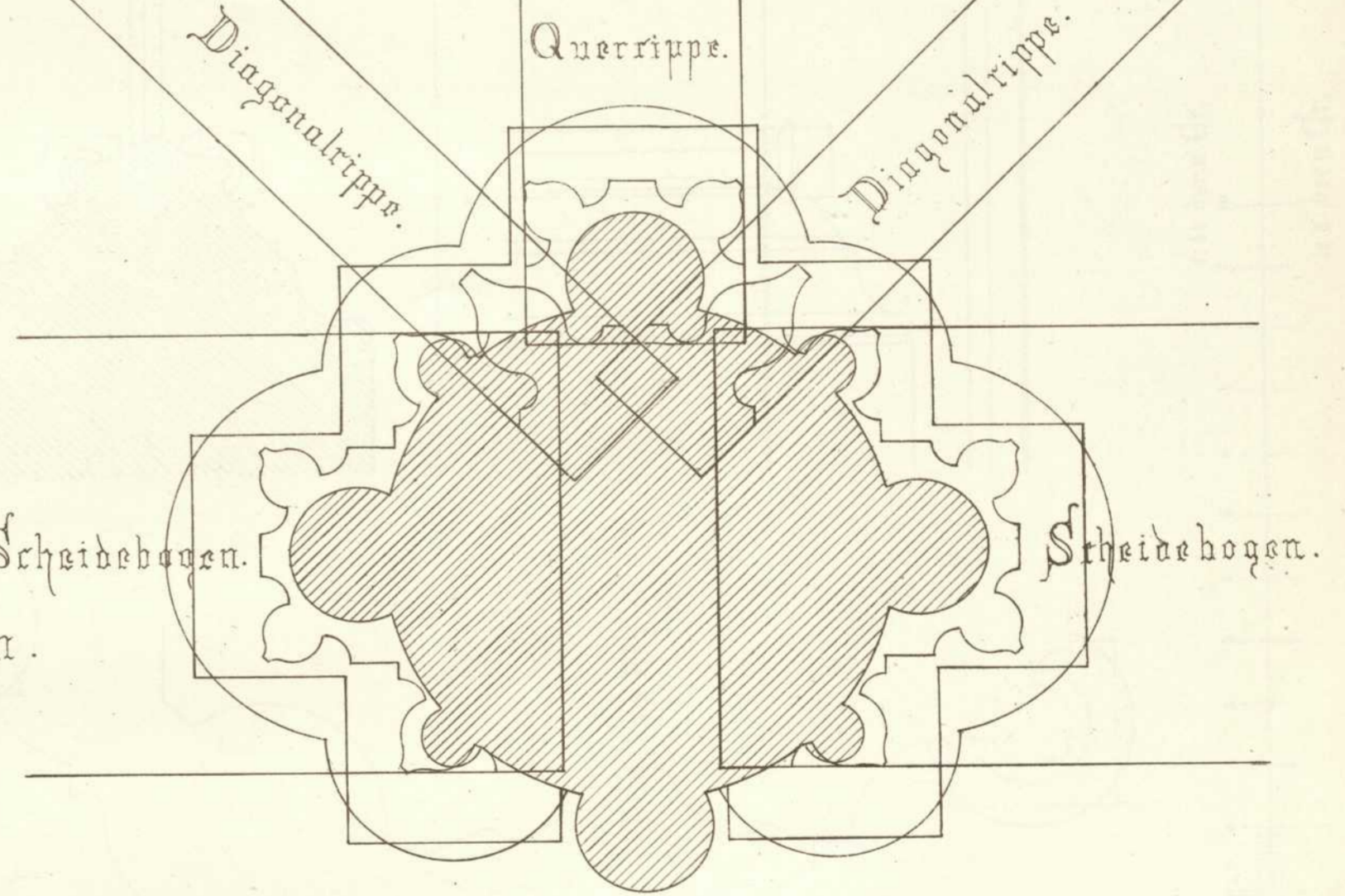
Grundriß der Gewölbanfänge des Seitenschiffes.
