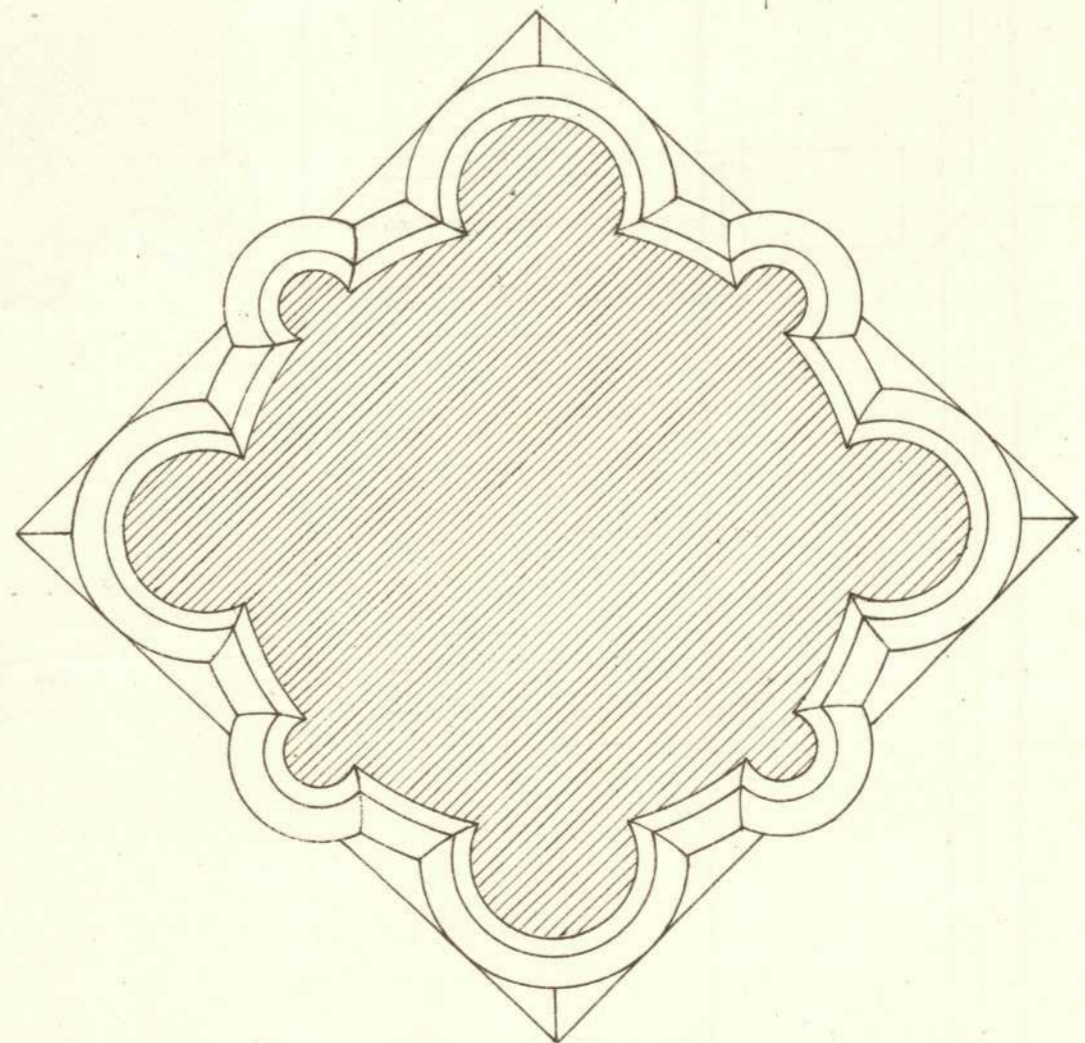
Grundriß des Pfeilerfußes.
