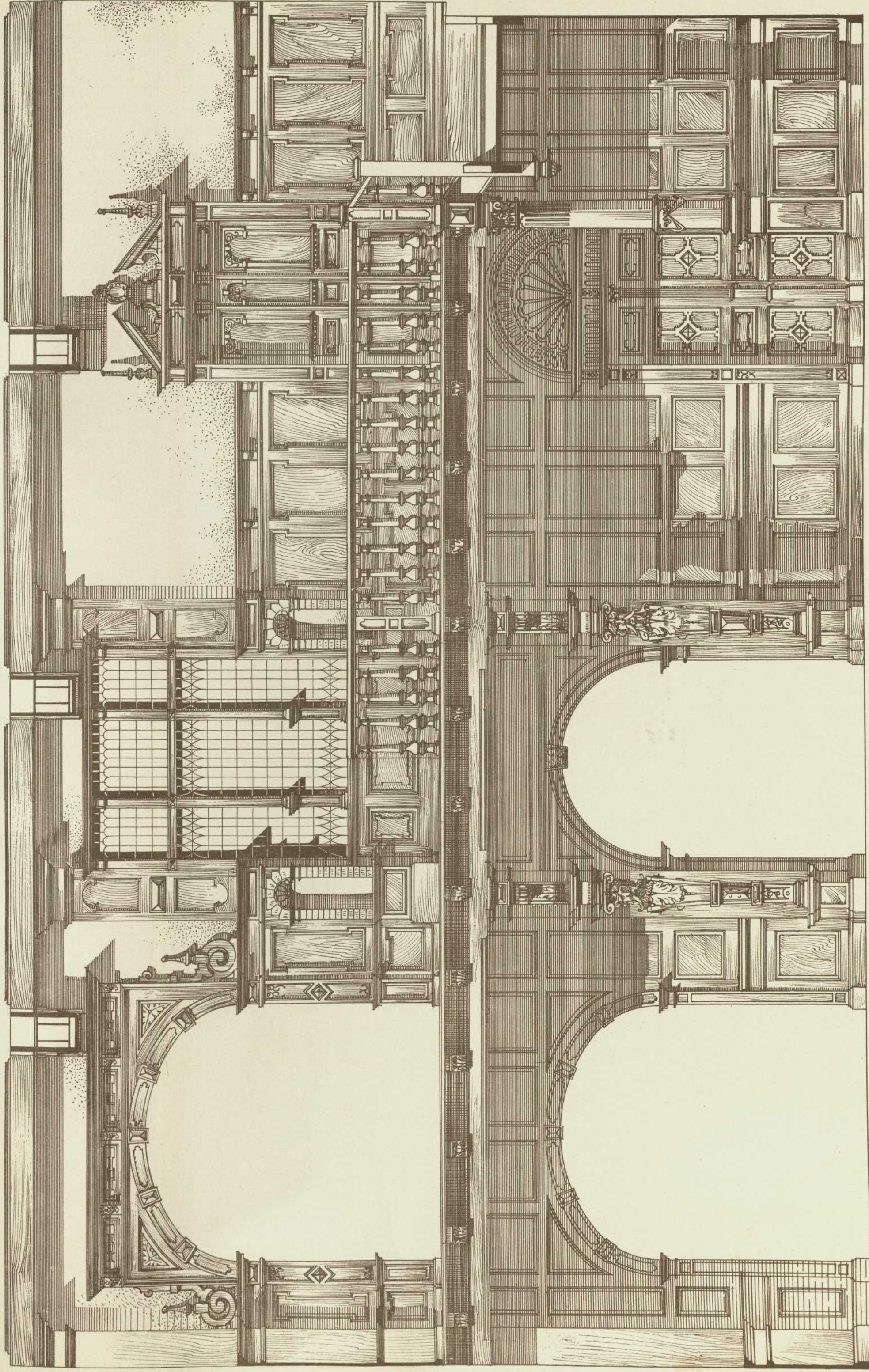
Schloss Wiesedonau Längenschnitt durch die Halle.
