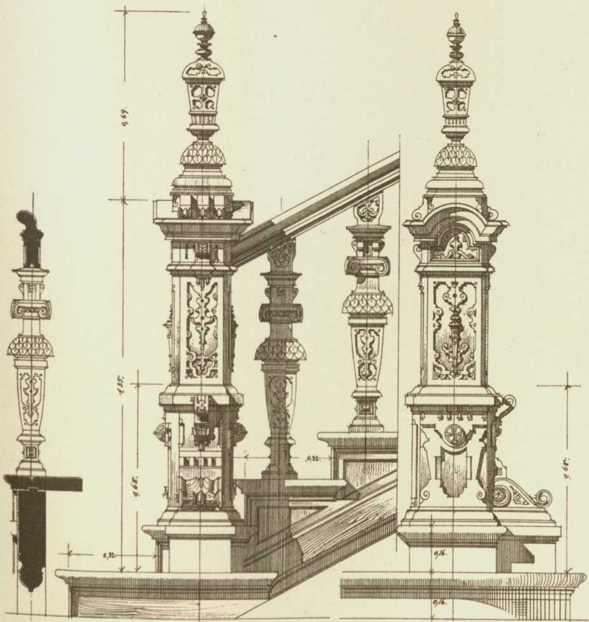
Treppe zum Speisesaal im Schlosse Bessedow - Arch: Prof. Dr. Haupt-Kannover.
