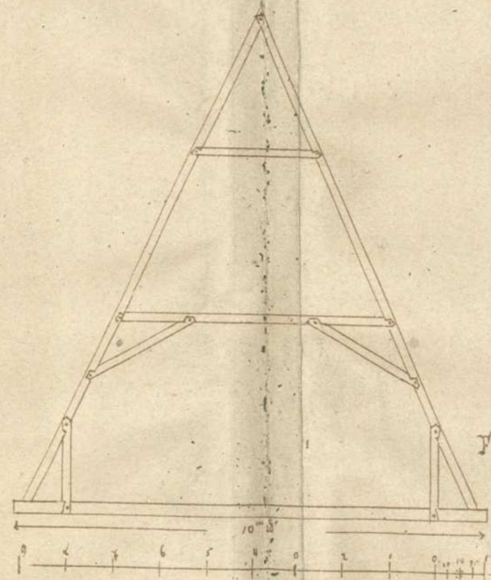
DACHSTUHL der
