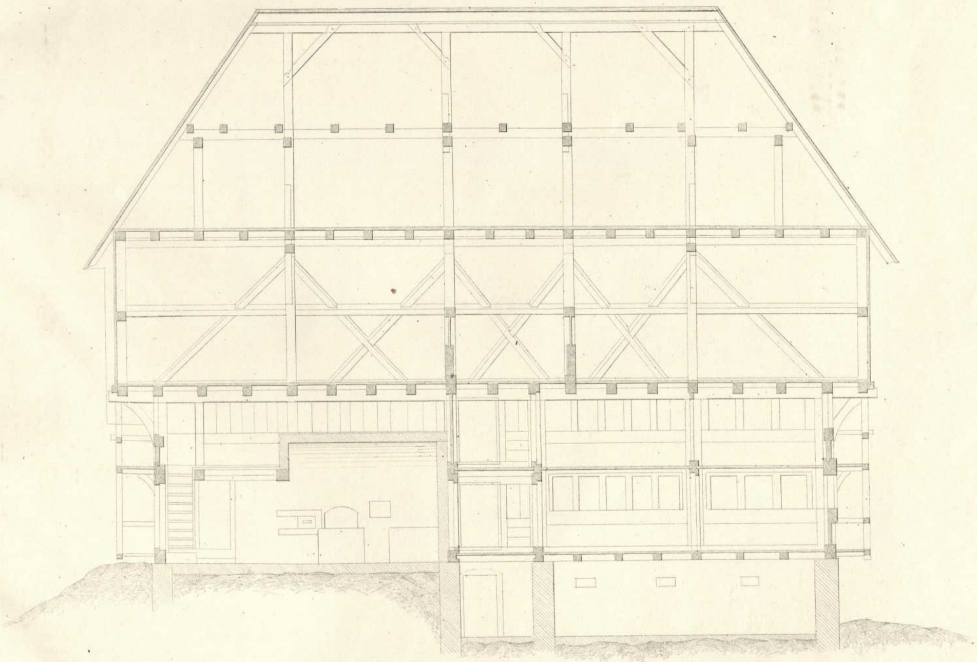
Schnitt nach yy.
