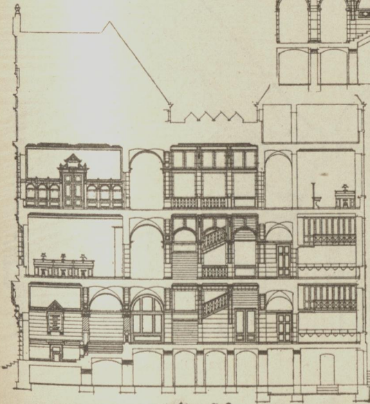
Schnitt A-B
