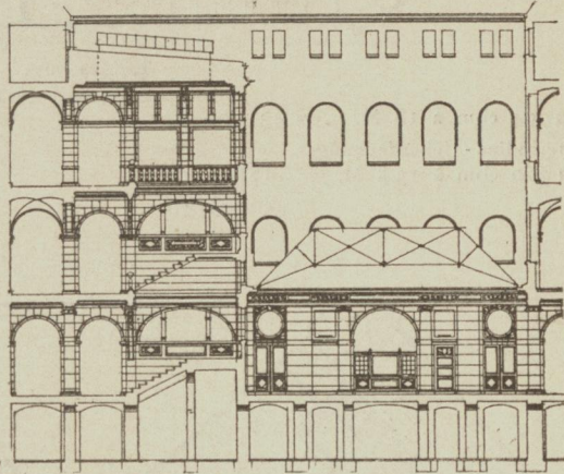
Schnitt C-D.
