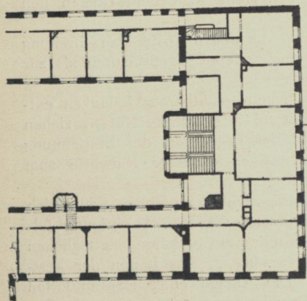
1. Obergeschoss.
