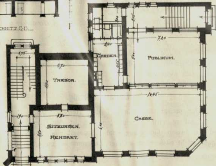
No. 1. (Kennwort: Ohne Ziegelrohbau.) 2. Preis. Giesecke & Wenzke-Charlottenburg.
