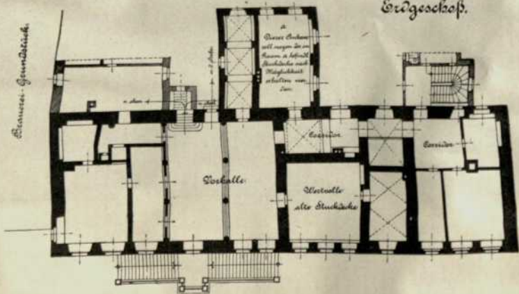
Grundrisse des alten Rathausbaues.
