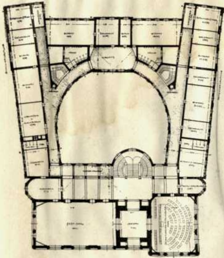
II. OBERGESCHOSS
