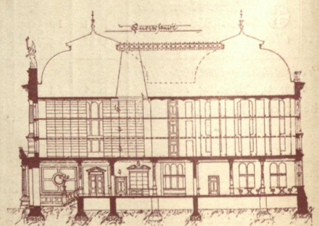
No. 1. Vorentwurf der Hochbau-Inspektion Bremen.
