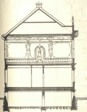
Querschnitt A-B durch den Kuppelgang
