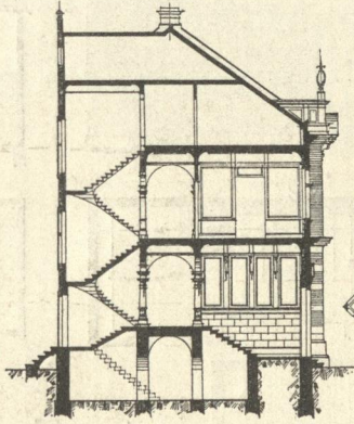
Querschnitt C-D durch den Treppengang
