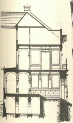
Querschnitt E-F durch den Treppengang
