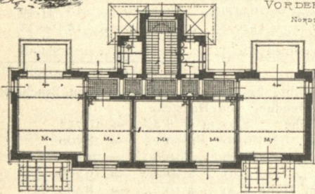
1. Obergeschoss.
