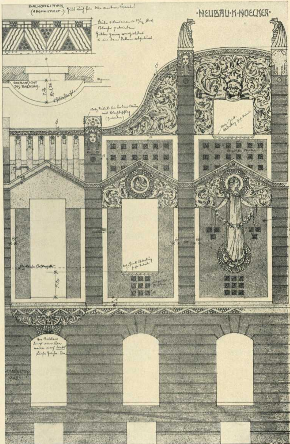
WOHN- UND GESCHÄFTSHAUS DETAIL
