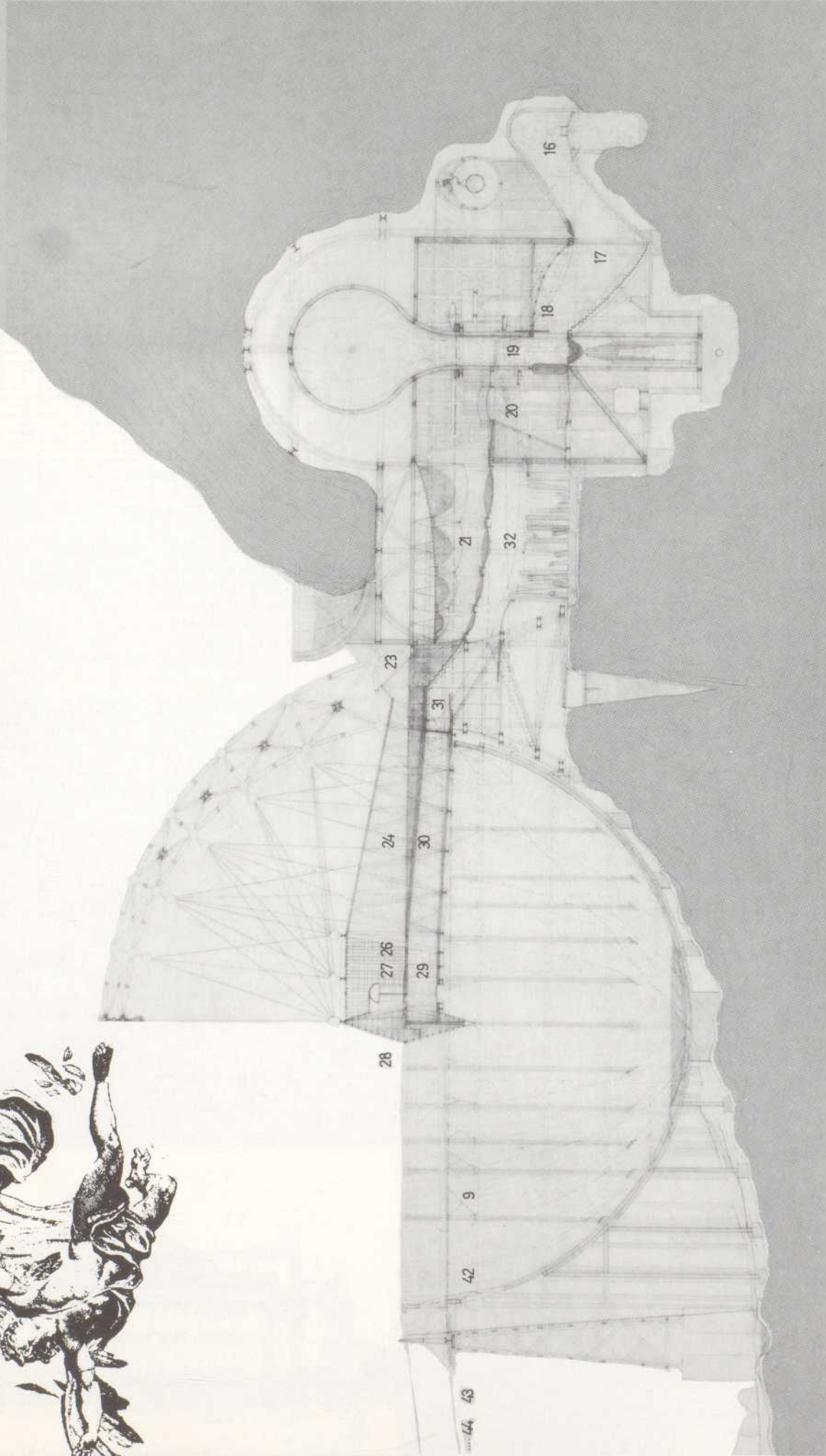
Längsschnitt: Bergstation
