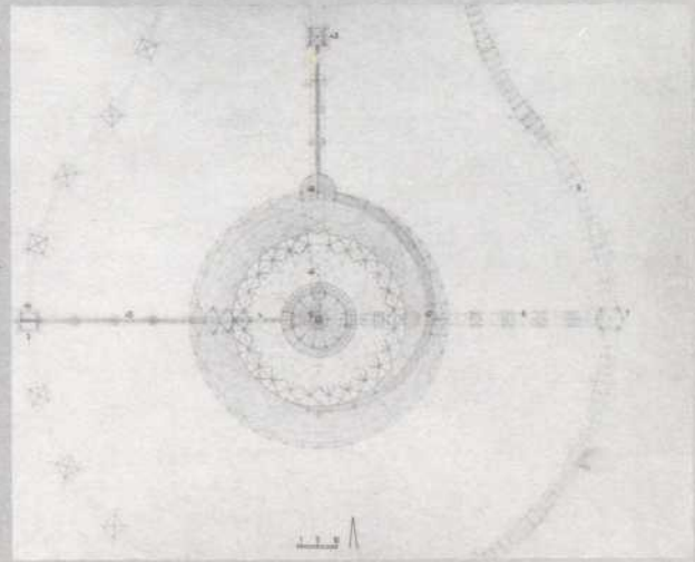
Grundriß: schwimmende Talstation
