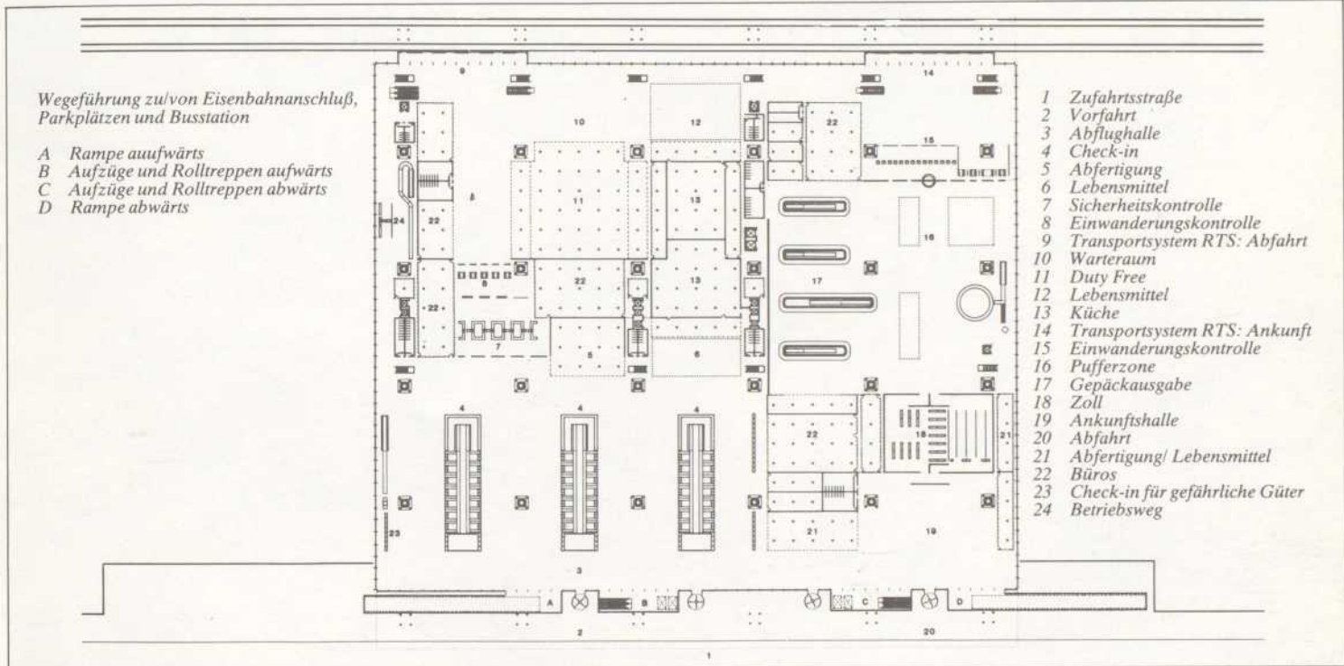
Grundriß Obergeschoß
