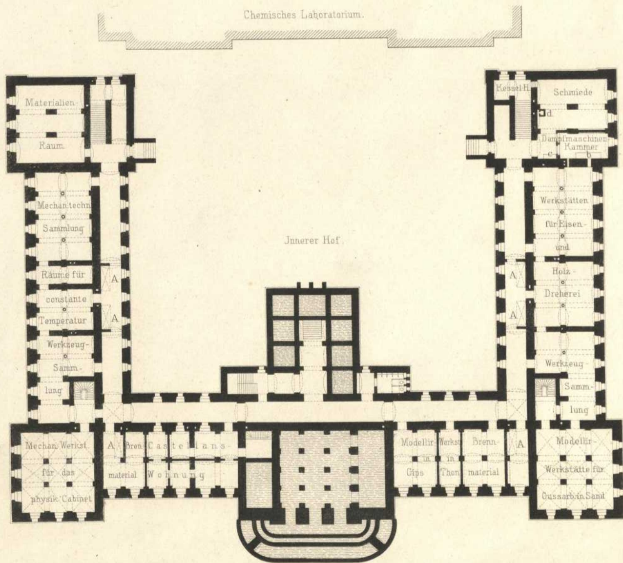
Grundrifs vom Souterrain.
