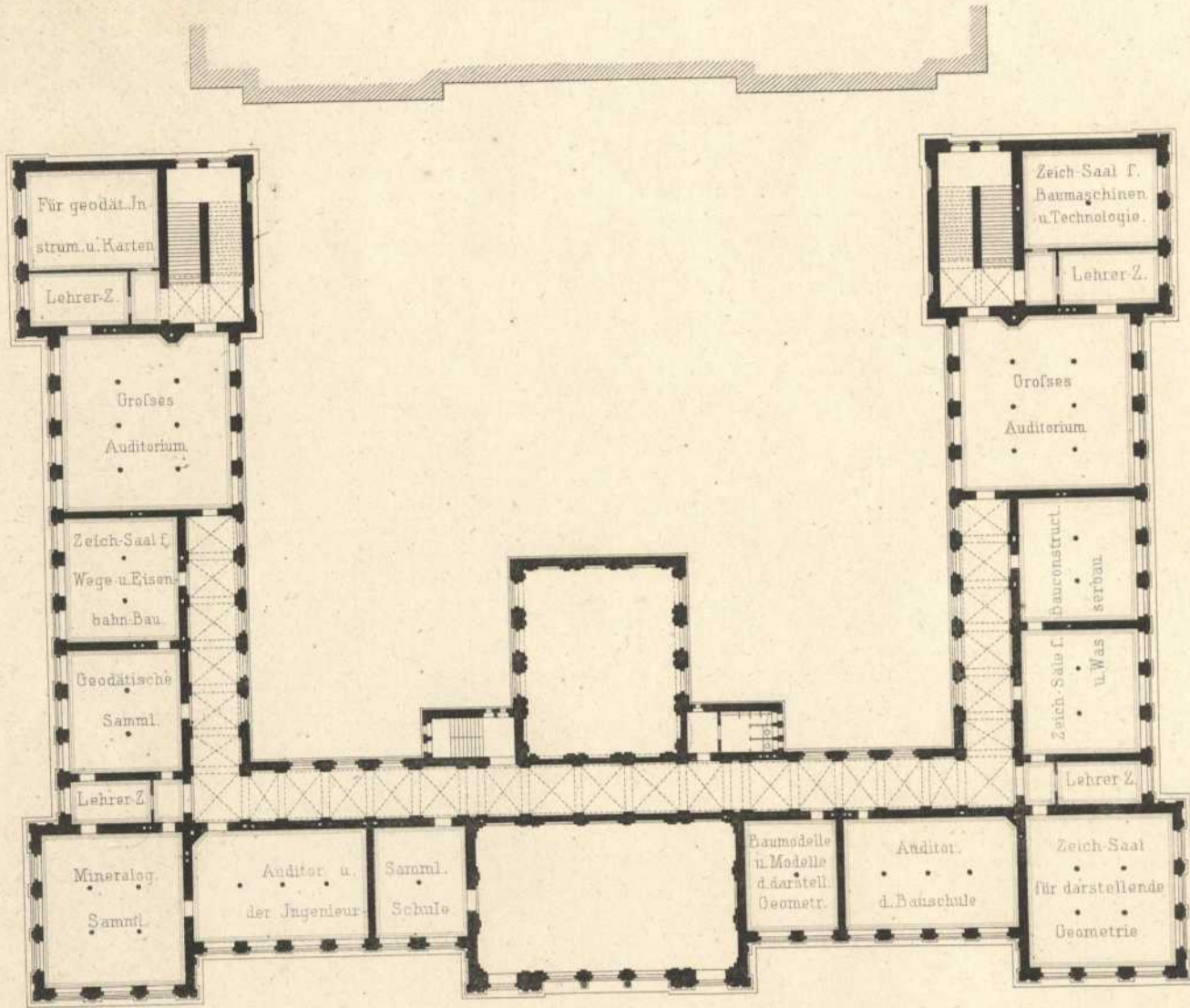
Grundriss vom 2ten Stock.
