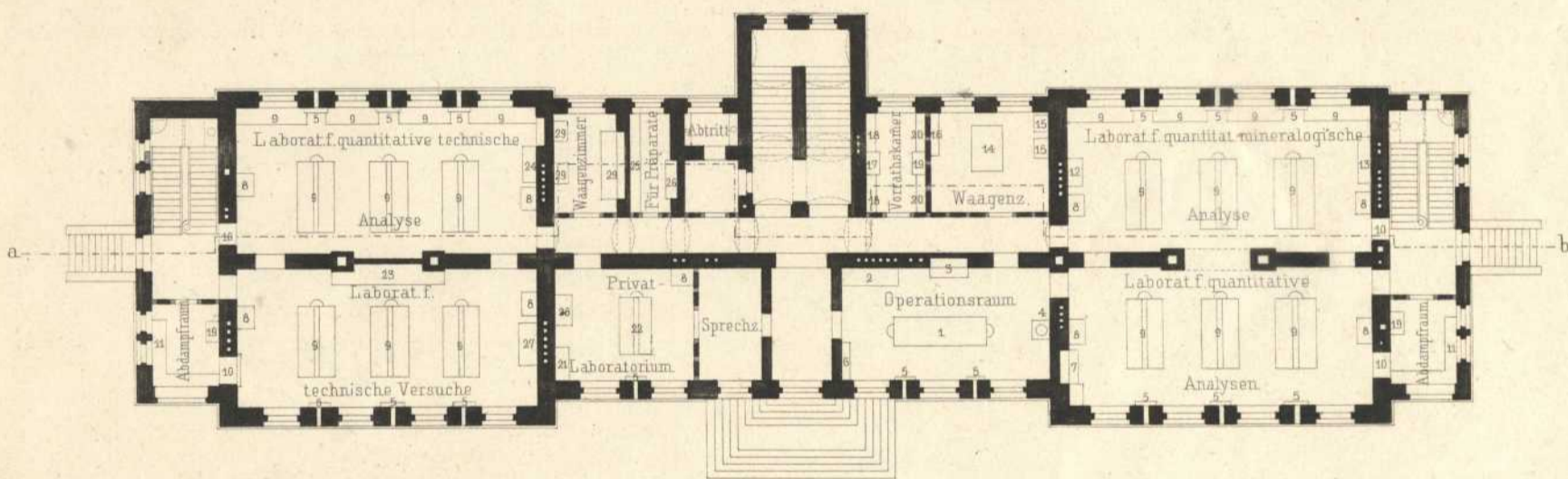
Grundriß vom Erdgeschofs.
