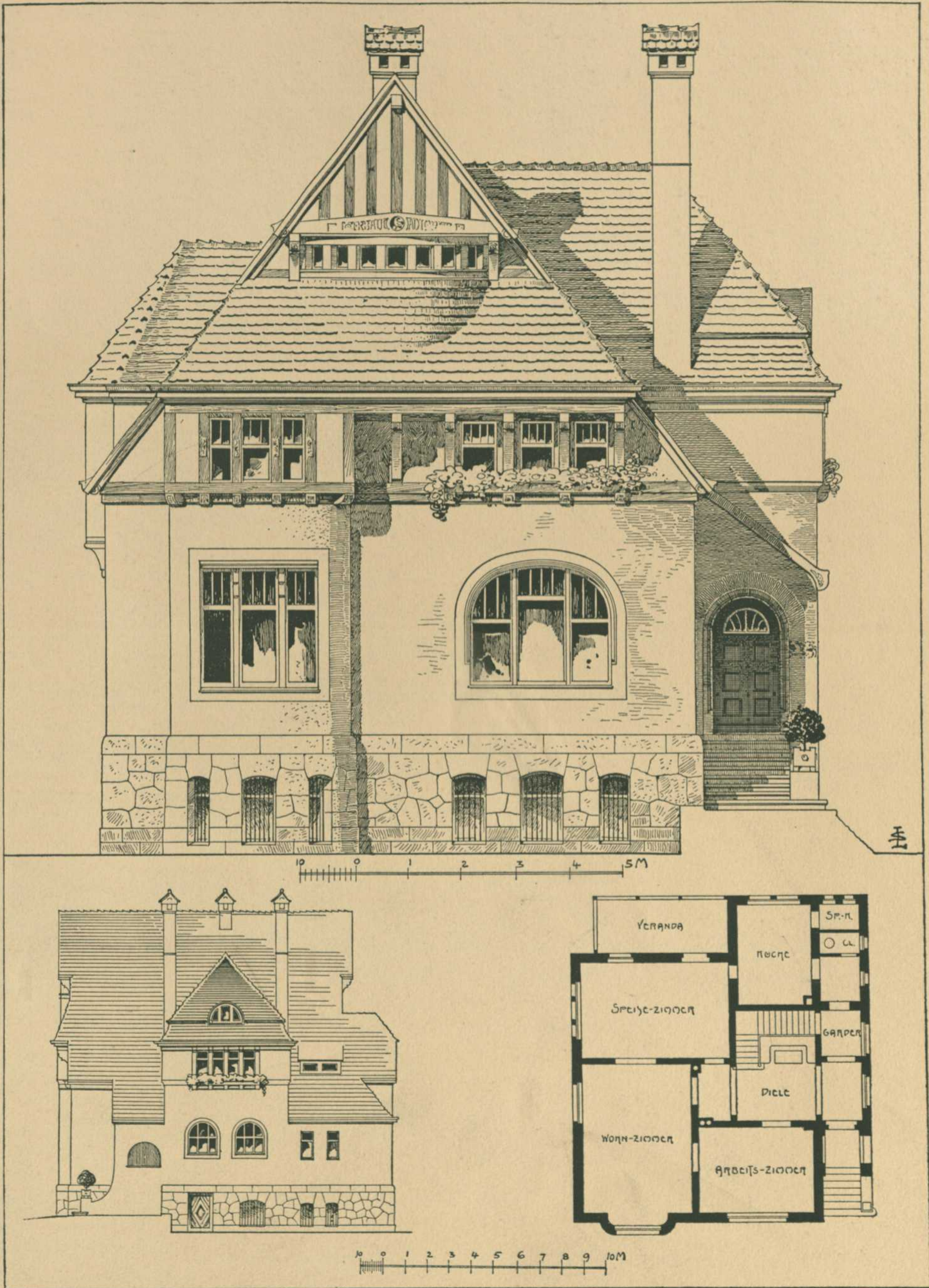
VILLA IN PLAUEN-DRESDEN. ARCHITEKT: PROFESSOR FRITZ SCHUMACHER IN DRESDEN.
