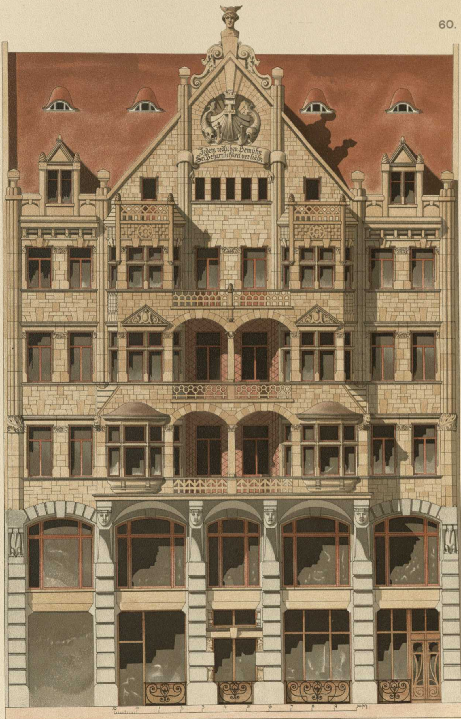
GESCHÄFTSHAUS IN LEIPZIG. ARCHITEKT: ALB. CONRAD IN LEIPZIG.
