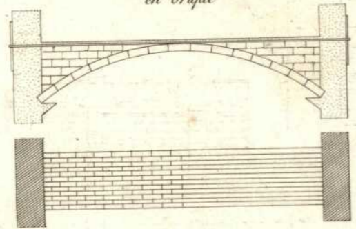
ou Voutes plates
