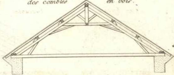
des combles en bois
