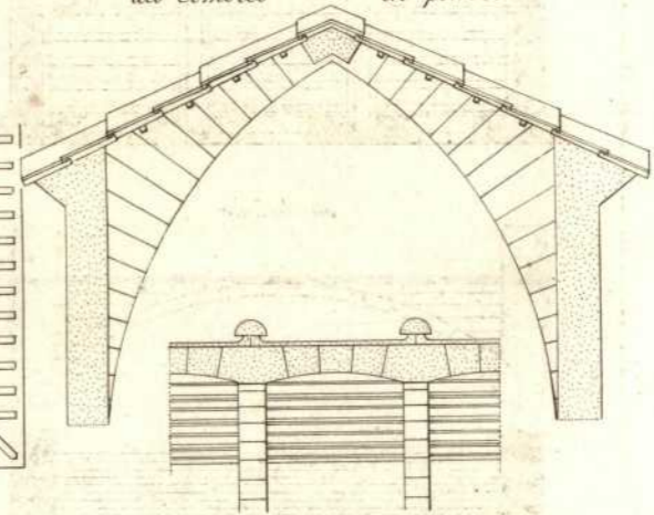
des Combles en pierres
