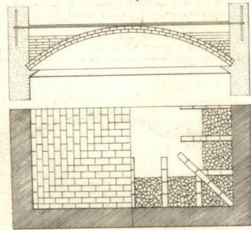
ou Voutes plates
