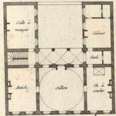
Etage
