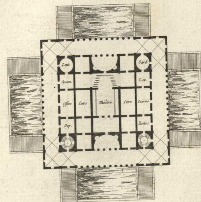
Souterrains
