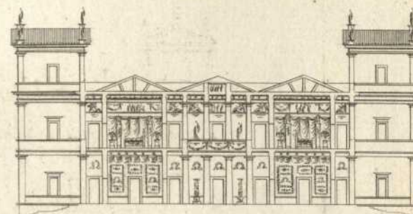
Coupe.
