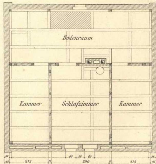
Halb - Geschoss.
