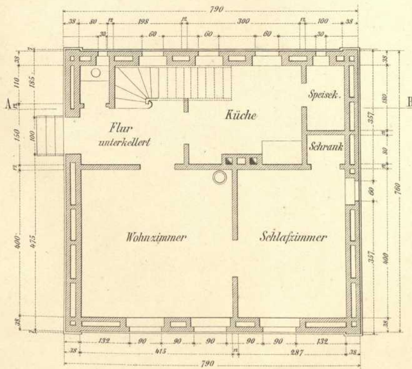
Erd - Geschoss.
