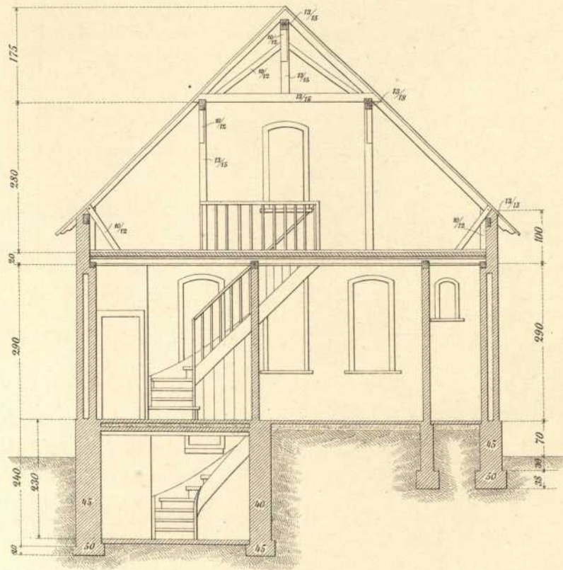
Halb - Geschoss.
