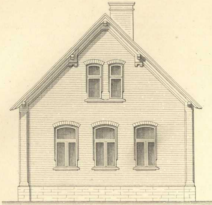
Giebel - Ansicht.
