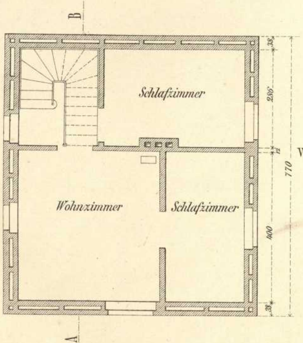
Ober-Geschoss.
