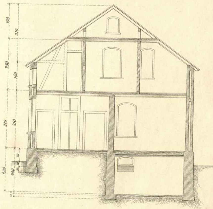
Schnitt C-D.
