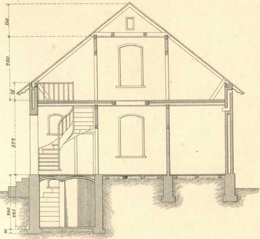
Halb-Geschoss.
