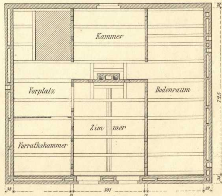
Halb-Geschoss.
