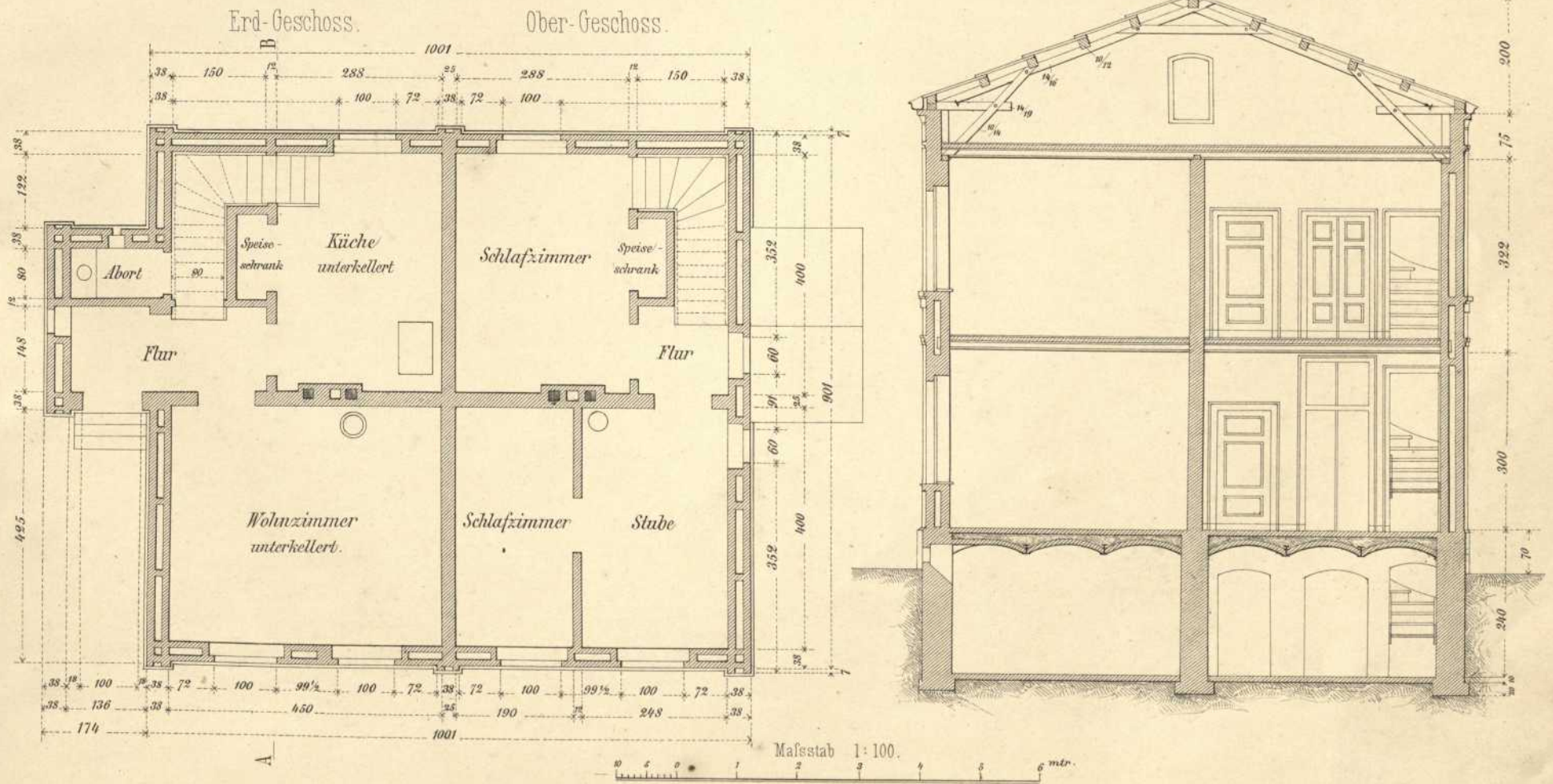
Schnitt A-B.
