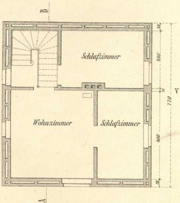
Ober-Geschoss.
