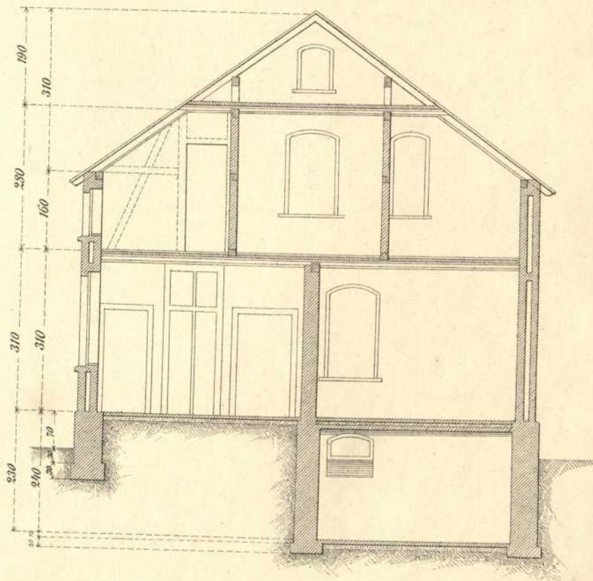
Schnitt C-D.
