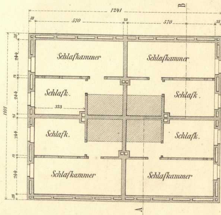
Dach-Geschoss.
