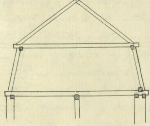
Leergesperr zu Fig. 179
