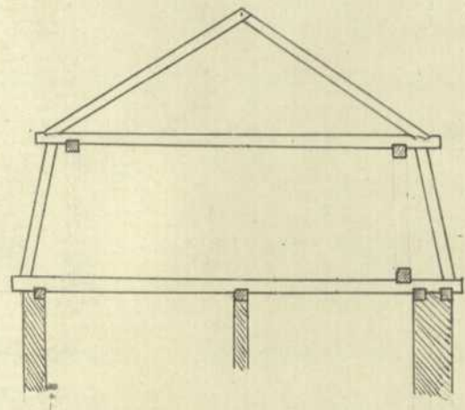
Leergesperr zu Fig. 178
